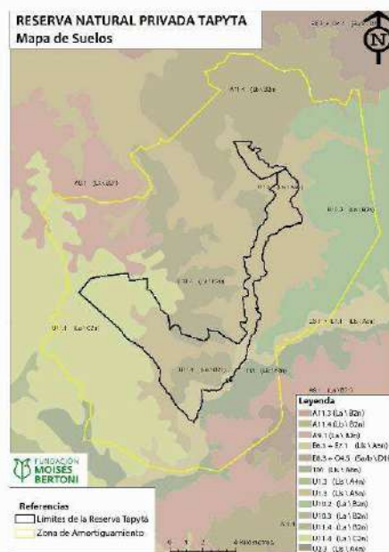
Mapa 12: Suelos
